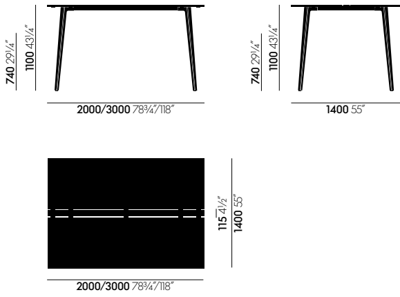
Joyn 2 Touchdown Tisch 200/300 x 140 cm, Tischhöhe 74/110 cm
